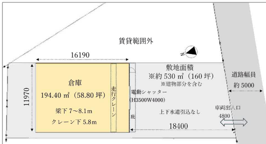
配置図・案内図
